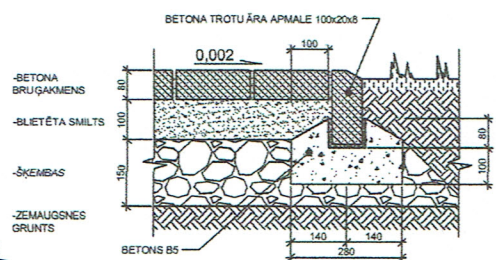
ŠKĒLUMS a-a
